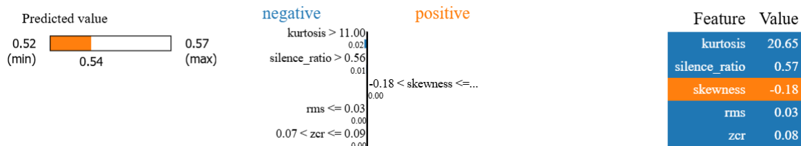
Figura 3.29: Explicación local energía Lime.
