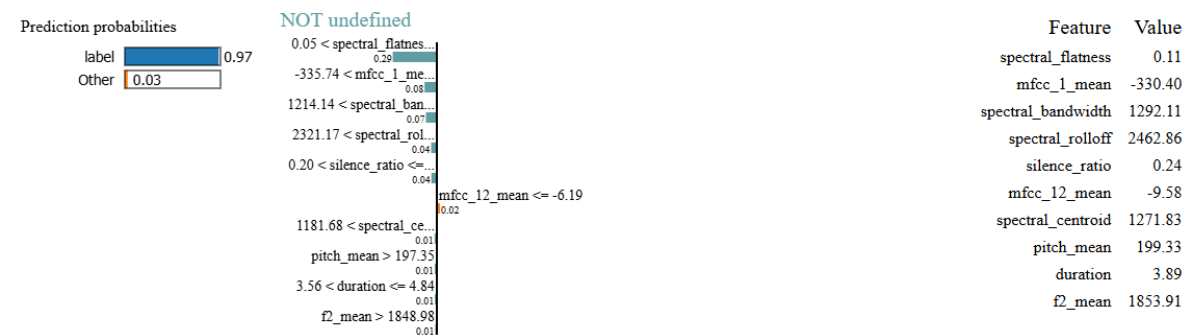
Figura 3.9: Explicación local con LIME
