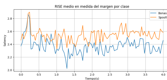
(b) Resultados de “margin” usando RISE.
