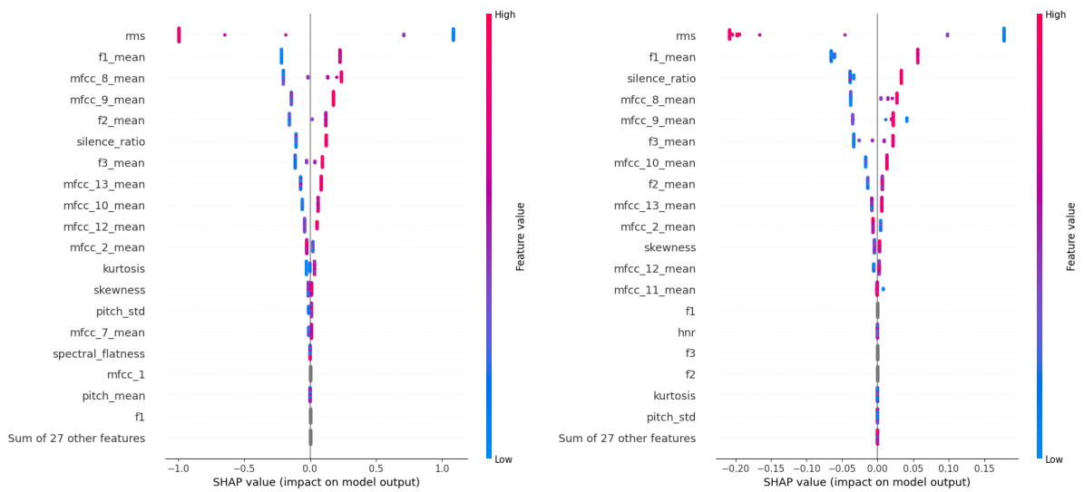
(a) Agrupación de las gráficas SHAP del clasifica- (b) Agrupación de las gráficas SHAP del regresor. dor.
